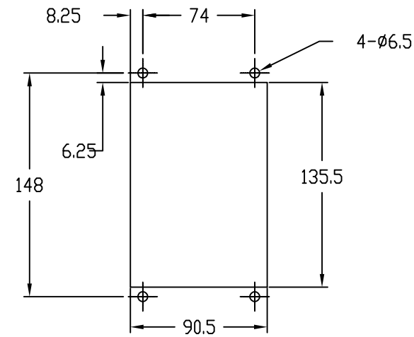
客户安装面板开孔尺寸
